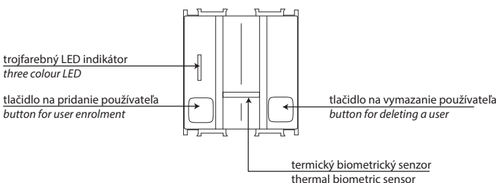
externá jednotka exterior unit
